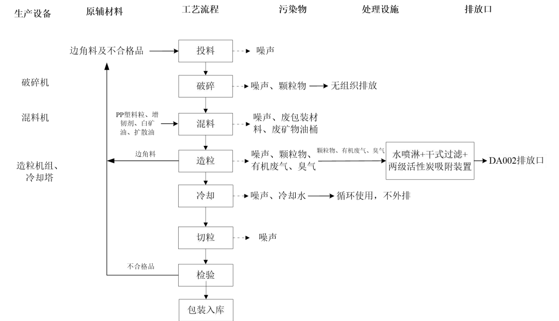
图2-5 改性塑胶粒生产工艺流程及产污环节示意图
