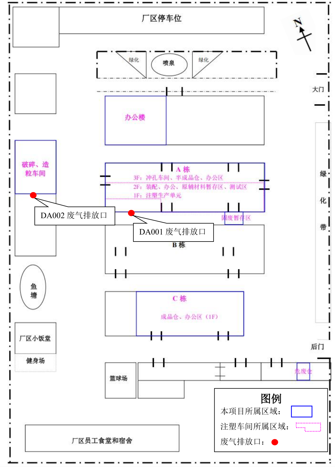
附图 2 项目厂区总平面图
