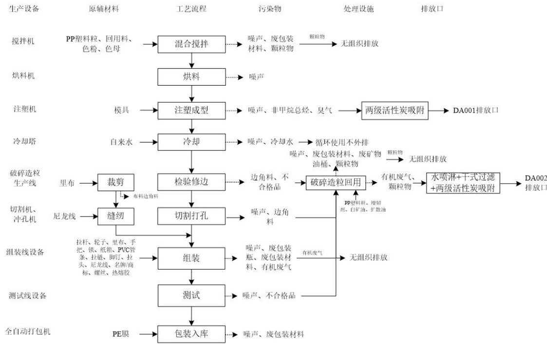
图 2-3 拉杆箱、塑料衣箱生产工艺流程及产污环节示意图
