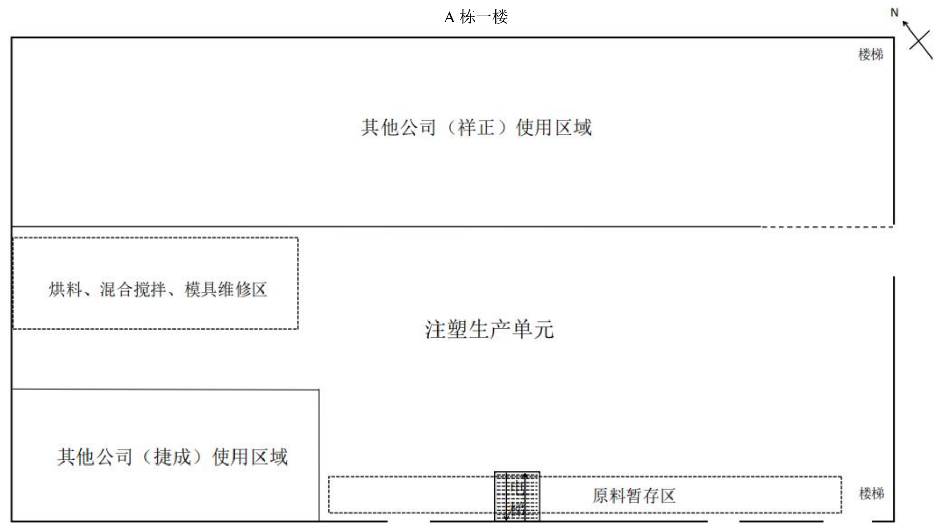
附图 4 项目车间平面布置图（A 栋）
