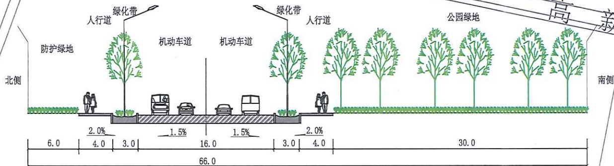
高新六路标准横断面 (K0+000~K0+240.000已铺设水泥路面)
